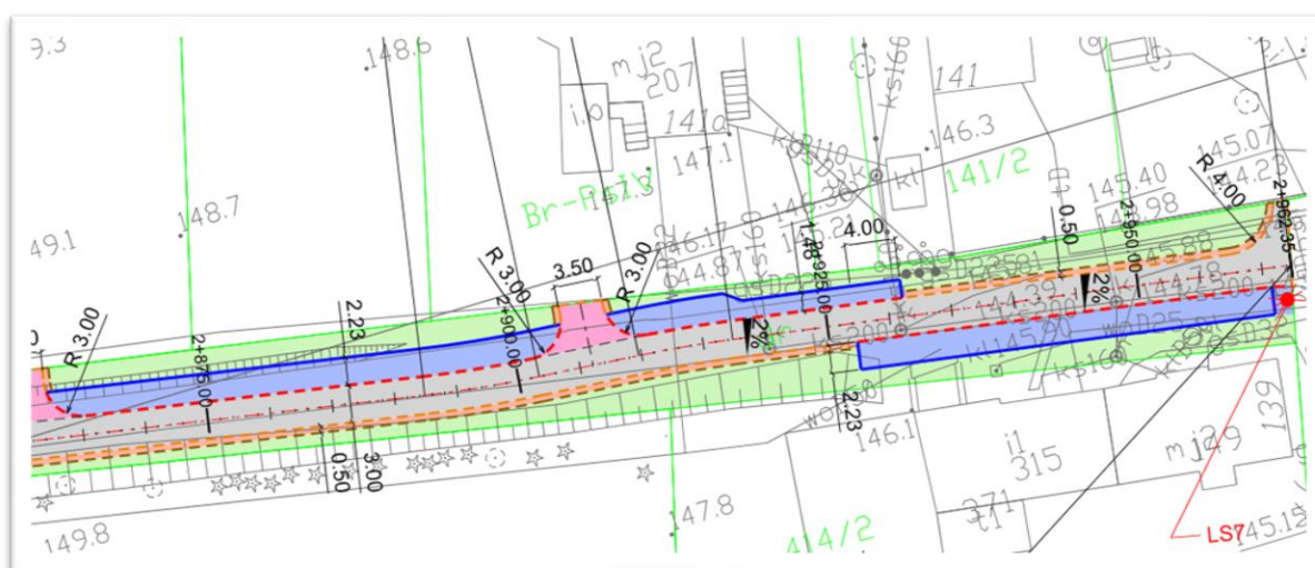
Rys. 1. Fragment projektu
